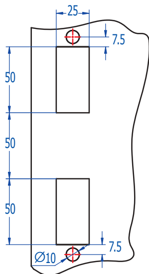
Dimensiones del orificio
