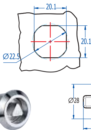
Dimensiones del orificio
