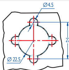
Dimensiones del orificio
