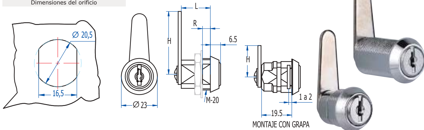
Dimensiones del orificio
