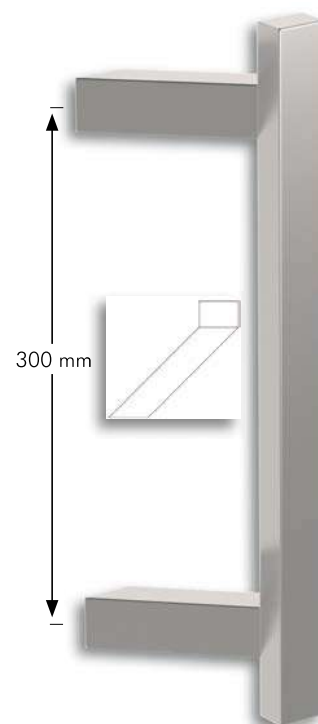
JÚPITER Largo 400 mm* 30x20 mm Ref: TJUP40- (simple) Ref: JTJUP40- (juego) (DESPLAZADO)
