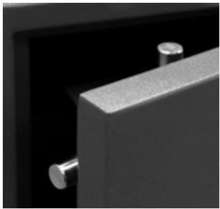
Cuerpo relleno de hormigón antivandálico con fibras de acero
